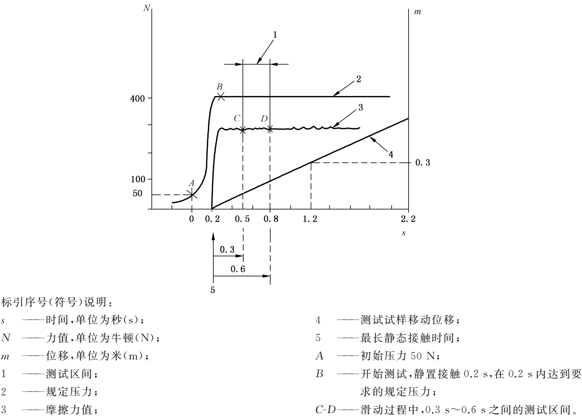
图 1 测试曲线图
